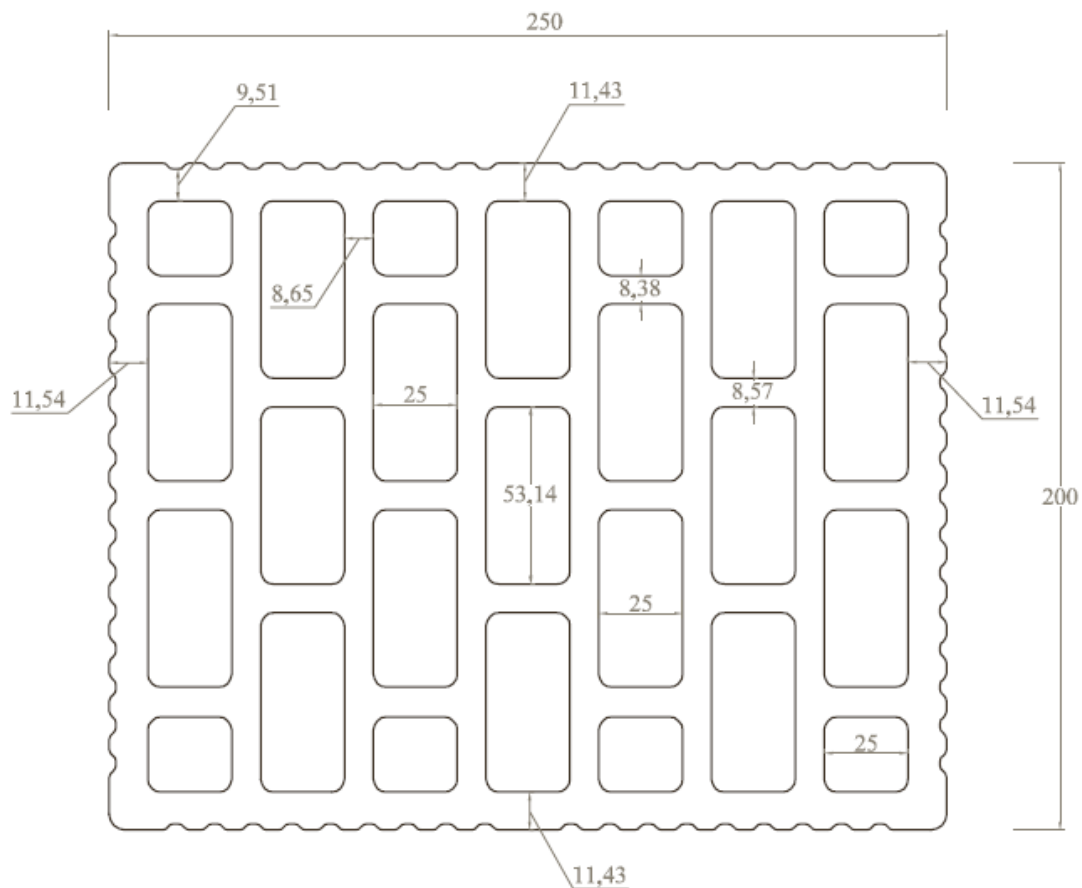
Σχήμα 1. Γεωμετρία οπτόπλινθου
